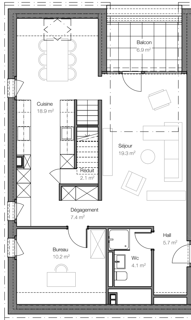
Etage 2
