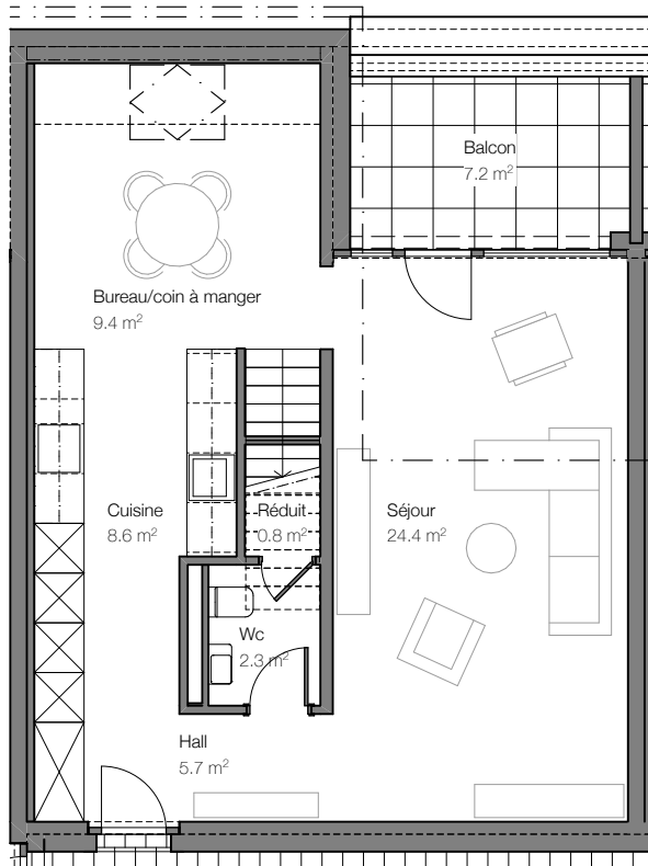
Etage 2
